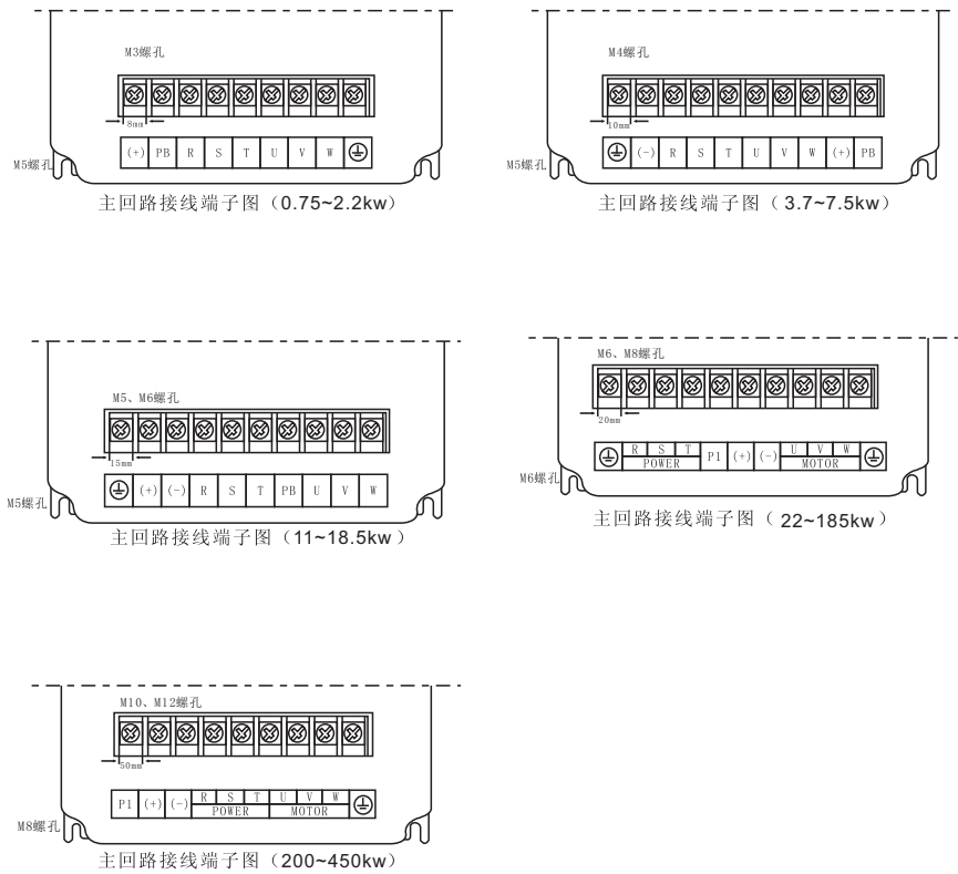
图3-14 变频器主回路端子分布
