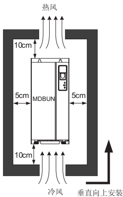
图2-9 VFDBU制动单元的安装间距
