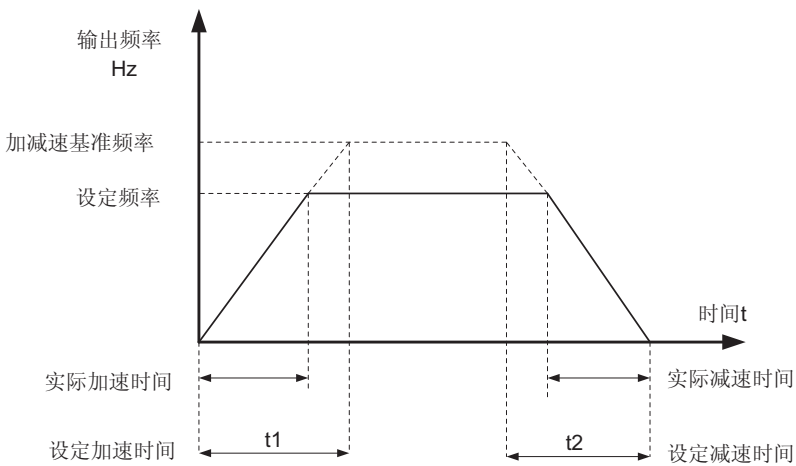
图5-21 加减速时间示意图
