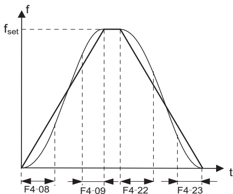
图5-24 S曲线加减速C示意图
