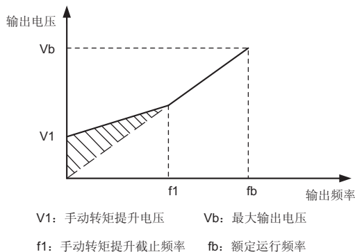
图5-34手动转矩提升示意图
