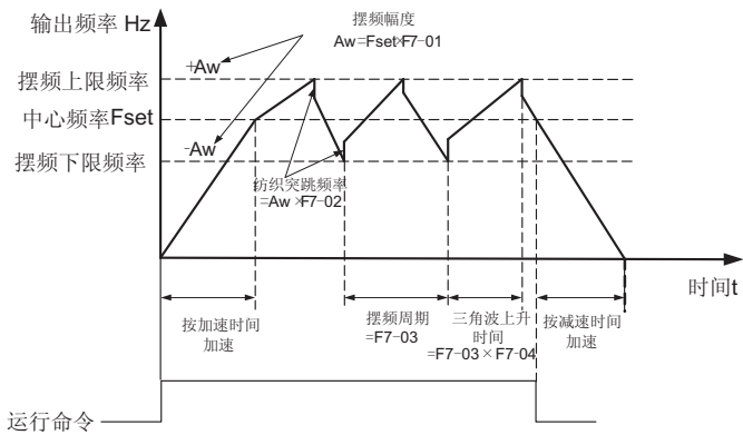
图5-45 摆频运行示意图
