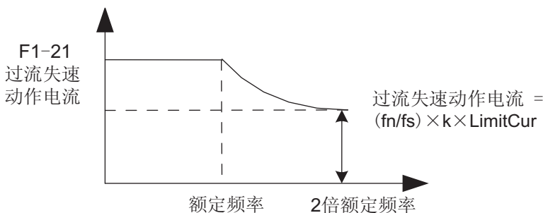
图5-36 倍速过流失速动作示意图
