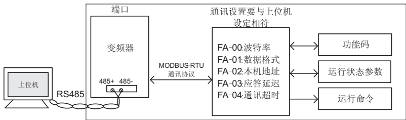
图3-24 变频器串行通讯的使用
