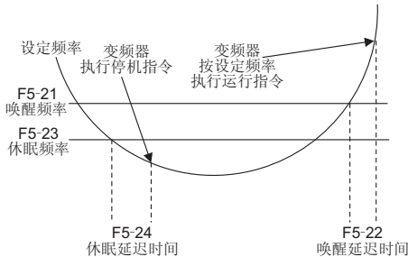
图5-44 休眠与唤醒延迟时间
